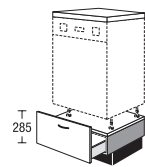
US 60 29 K1GS Modulschrank für hochgebaute Geschirrspüler Modular unit for raised dishwasher
