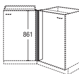
UPEF135 87 Eckpassleiste für 135° Eckeinbau von Unterschrank Corner infill panel for 135° base unit corner installations
