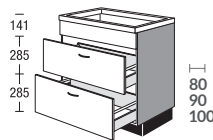
KDB2A ... Kochstellenschrank für Muldenlüfter Hob base unit for hob extractor
