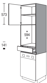
CABS 139 H Aufsatzschrank als Aufsatzschrank auf E-Geräte Top unit as top unit on electrical appliances
