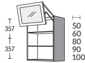
CHFKGU ... 02 N1 Hängeschränk mit Falttür Wall unit with folding door
