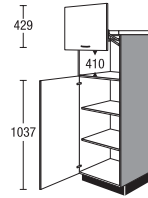
GM 148 L5 Highboard für Einbaugeräte mit Lifttür Highboard for built-in appliances with lift-up door
