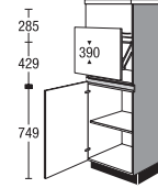
CGM 151 HL Highboard für Einbaugeräte mit Lifttür Highboard for built-in appliances with lift-up door
