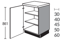
U ... FV Unterschrank Base unit
