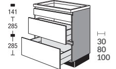
CKDB2A ... Kochstellenschrank für Muldenlüfter Hob base unit for hob extractor
