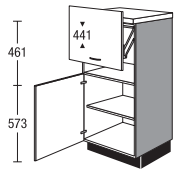
GM 104 LX Highboard für Einbaugeräte mit Lifttür Highboard for built-in appliances with lift-up door
