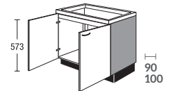
SP ... 58 Spülen-Unterschrank 579 mm hoch Sink base unit, 579 mm high
