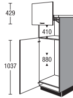
G88M 148 L5 Highboard für Einbaugeräte mit Lifttür Highboard for built-in appliances with lift-up door
