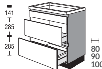
CSPB2A ... SK2 Spülen-Unterschrank für Quooker Systeme Sink base unit for Quooker systems
