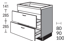
SPB2A ... SK2 Spülen-Unterschrank für Quooker Systeme Sink base unit for Quooker systems
