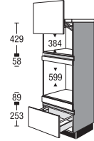
CGMBA 151 HL5 Highboard für Einbaugeräte mit Lifttür Highboard for built-in appliances with lift-up door
