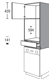
CABS 124 H Aufsatzschrank als Aufsatzschrank auf E-Geräte Top unit as top unit on electrical appliances
