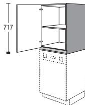
CA 60 78 H Aufsatzschrank als Aufsatzschrank auf E-Geräte Top unit as top unit on electrical appliances
