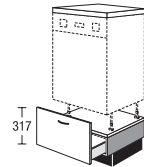
US 60 32 K1GS Modulschrank für hochgebaute Geschirrspüler Modular unit for raised dishwasher
