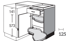
EKIS ... LMP EKIS ... LM Eck-Kochstellenschrank Corner hob base unit
