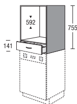
ABS 75 Aufsatzschrank für Backofen Top-mounted unit for oven
