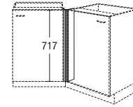
UPEF135 Eckpassleiste für 135° Eckeinbau von Unterschrank Corner infill panel for 135° base unit corner installations
