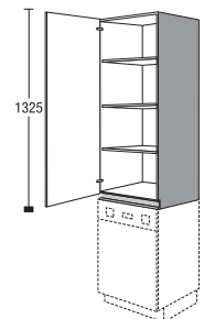
CA 60 139 H Aufsatzschrank als Aufsatzschrank auf E-Geräte Top unit as top unit on electrical appliances
