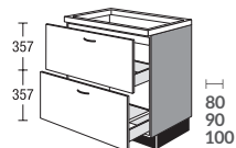
SP2A ... SK2 Spülen-Unterschrank für Quooker Systeme Sink base unit for Quooker systems
