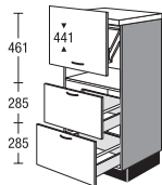
GM2A 104 LX Highboard für Einbaugeräte mit Lifttür Highboard for built-in appliances with lift-up door
