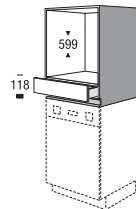
CABS 78 H Aufsatzschrank als Aufsatzschrank auf E-Geräte Top unit as top unit on electrical appliances
