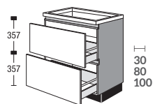
CKD2A ... CKD2A ... S Kochstellenschrank für Muldenlüfter Hob base unit for hob extractor
