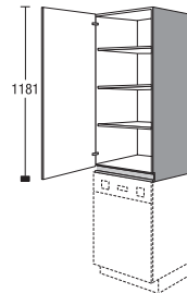
CA 60 124 H Aufsatzschrank als Aufsatzschrank auf E-Geräte Top unit as top unit on electrical appliances
