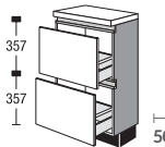
CU2A ... 79 33 Unterschrank mit Servosoft / Pro Servosoft Base unit with Servosoft / Pro Servosoft
